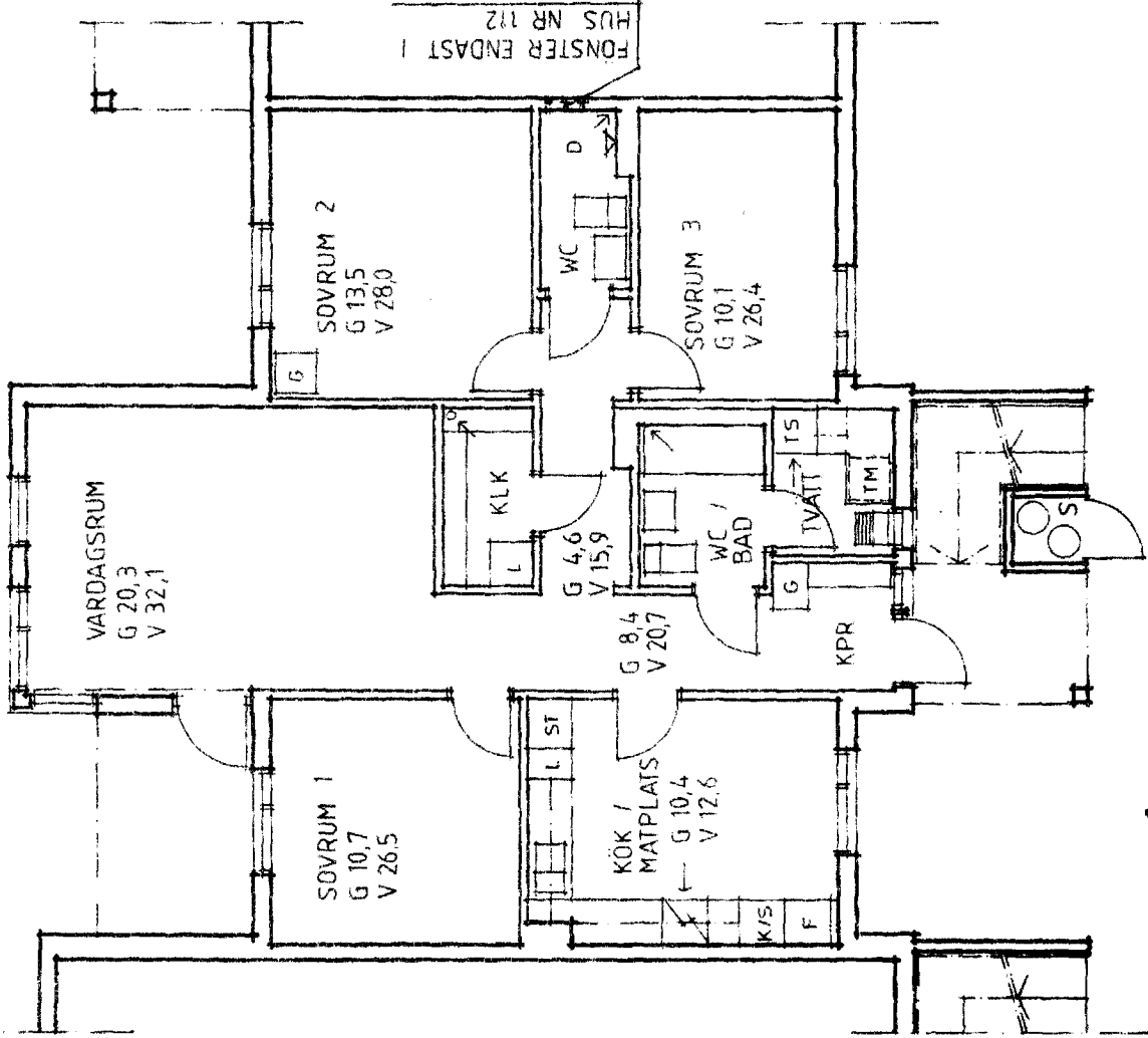
PLAN 1, 1:100
